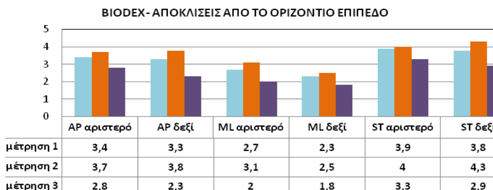
Σχήμα 1. Μέσες τιμές των αποκλίσεων από το οριζόντιο επίπεδο στους δείκτες: AP, ML, ST του Biodex Balance System, κατά τη μέτρηση 1, 2 και 3 με πόδι στήριξης: αριστερό-δεξί.
