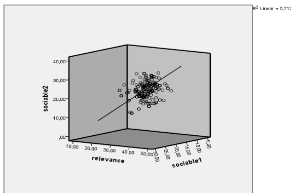
Σχήμα 1. Συσχετίσεις μεταβλητών
